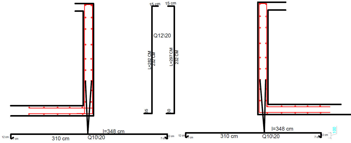
F-F kesiti donatı şeması
